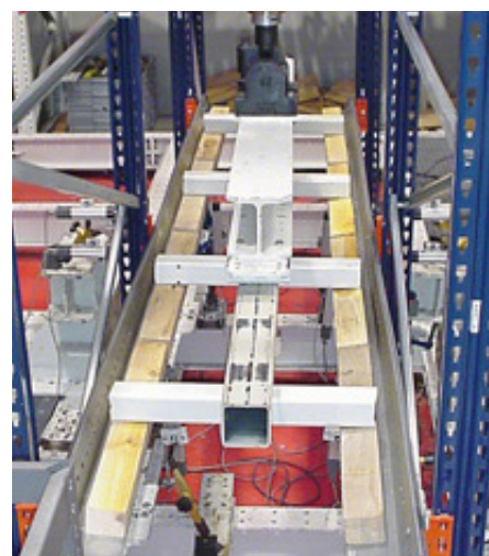
Ejemplo de ensayo de carril para paletización compacta
